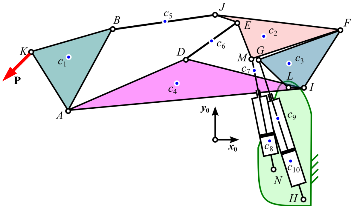
Rysunek 1. Schemat kinematyczny mechanizmu
